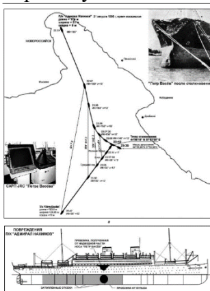
Рис. 1.4. Столкновение т/х «Петр Васёв» и т/х «Адмирал Нахимов»: а — траектории движения; б — столкновение парохода «Адмирал Нахимов»
